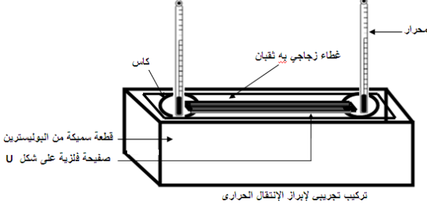
تركيب تجريبي لإبراز الإنتقال الحراري
